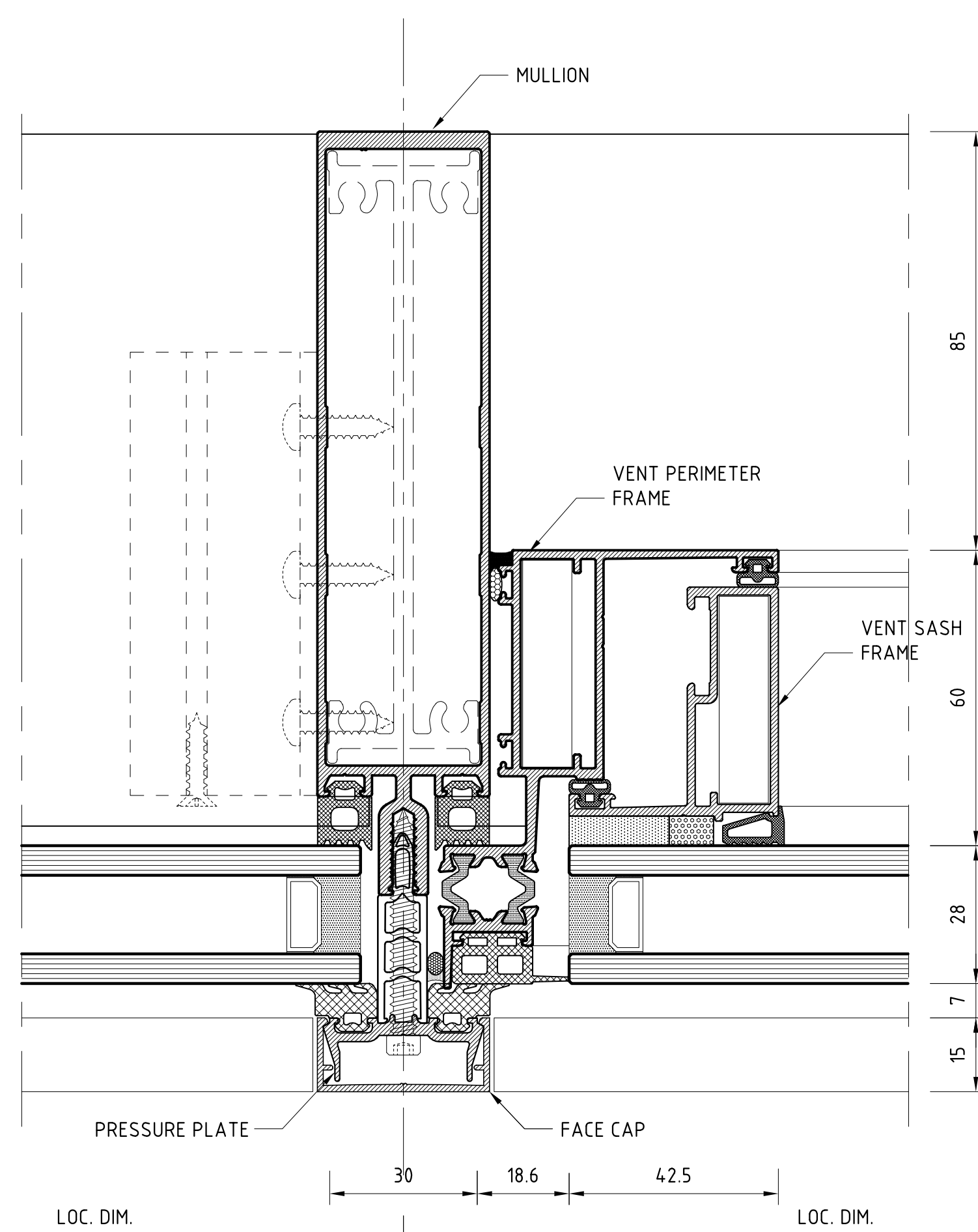
JAMB MULLION DETAIL
